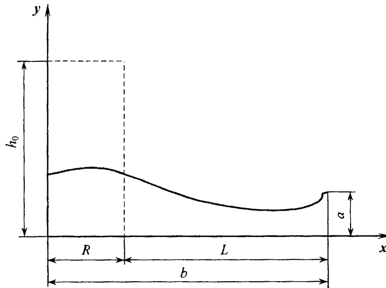
Рис. ПЗ.2. Типичная картина движения жидкости в обваловании при квазимгновенном разрушении резервуара - - - - - уровень начального столба жидкости; ———— - уровень жидкости в промежуточный момент времени (результаты расчета)
